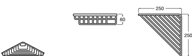
Nuova 816534001 Угловой контейнер-решетка.
