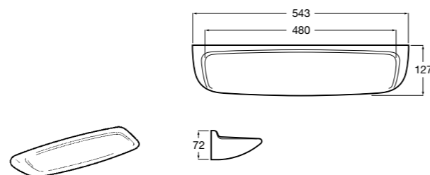
Onda Plus 380247001 Полочка.
