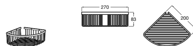
Hotel's 816731001 Угловой контейнер-решетка.
