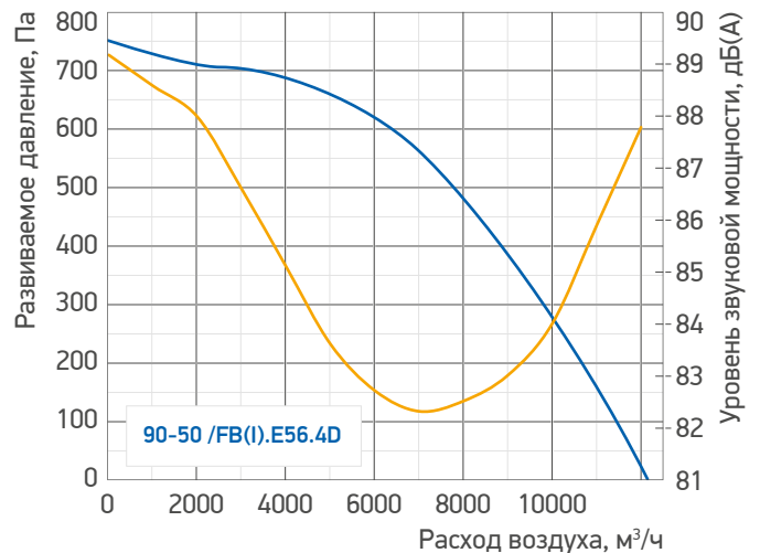
Гр. 14. Аэродинамические и звуковые характеристики вентиляторов /FB(I).E56.4D
