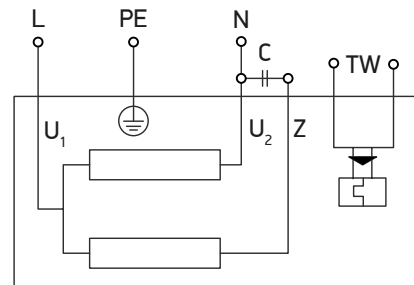
Схема 52. Схема подключения агрегатов воздушного отопления LM VEKTOR
