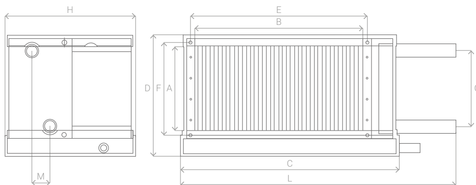
Схема 22. Габаритные размеры водяных охладителей /CW
