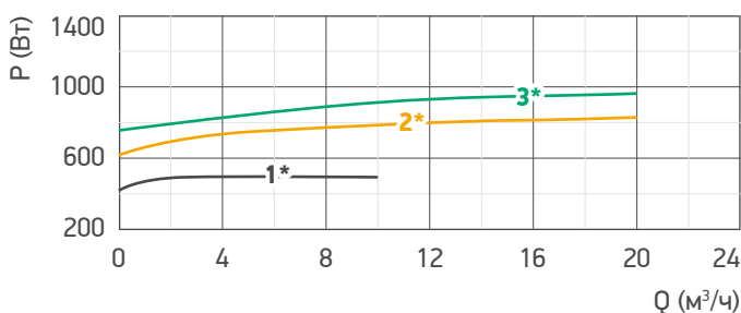
Гр. 74. Гидравлические характеристики насоса /P.3F.40H
