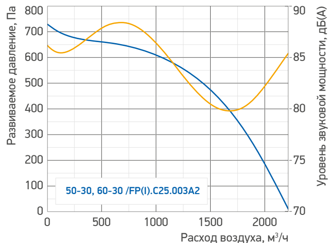
Гр. 2. Аэродинамические и звуковые характеристики вентиляторов /FP(I).C25.003.A2
