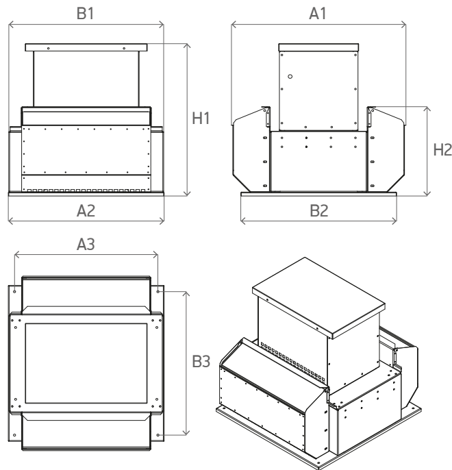
Схема 55. Габаритные характеристики вентиляторов /FPV
