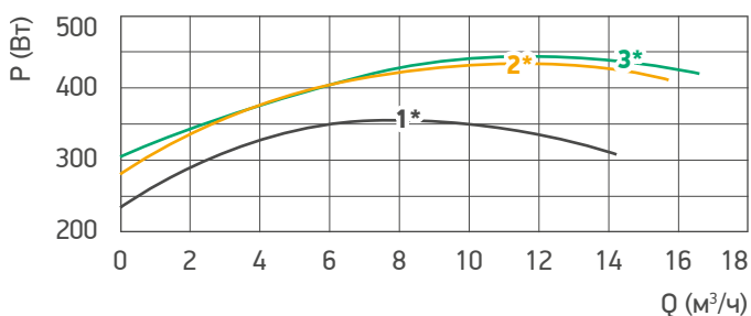
Гр. 73. Гидравлические характеристики насоса /P.1F.50
