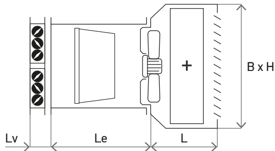
Схема 51. Габаритные характеристики агрегатов воздушного отопления LM VEKTOR
