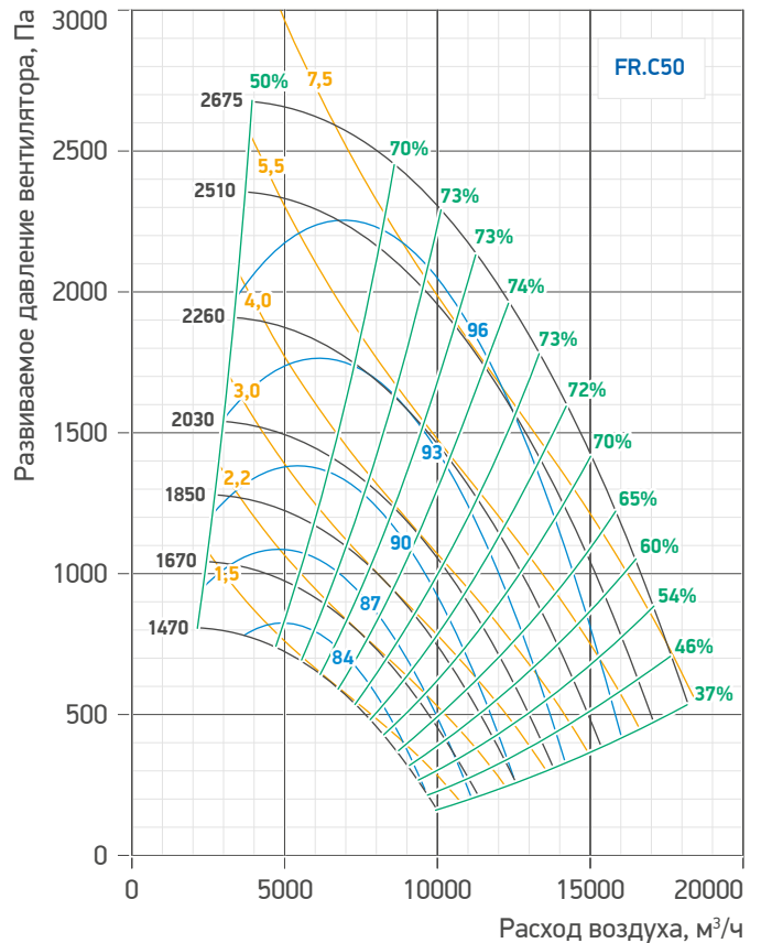
Гр. 58. Аэродинамические характеристики FR.C50
