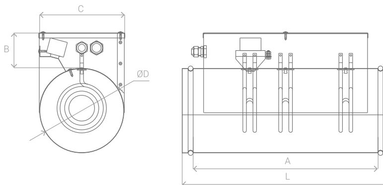
Схема 43. Габаритные размеры электрических нагревателей /HE
