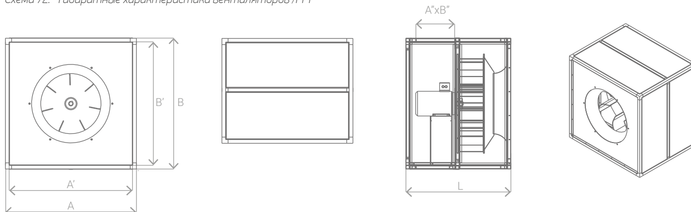
Схема 72. Габаритные характеристики вентиляторов /FPI
