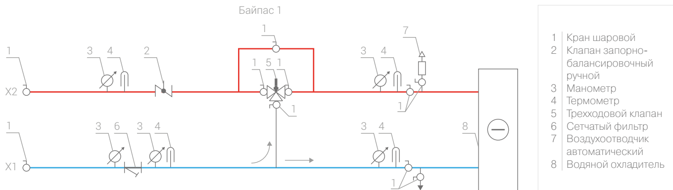
Схема 75. Схема обвязки охладителя водяного CW
