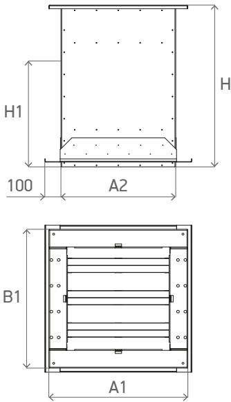
Табл. 55. Габаритные и присоединительные размеры монтажных стаканов /TSS._
