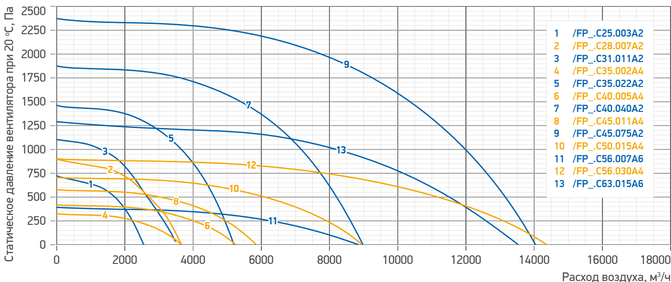
Гр. 42. Аэродинамические характеристики вентиляторов LM SAUGER /FP_ (продолжение)
