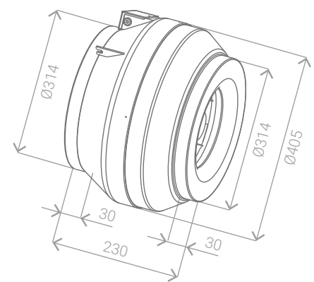
Схема 37. Вентилятор 315 /FBP.E28.2E
