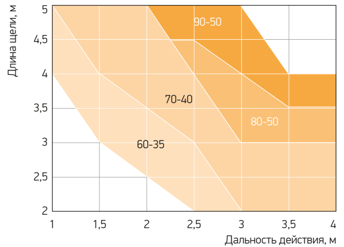
Гр. 40. Подбор воздушных завес по типу вентилятора. Стандарт
