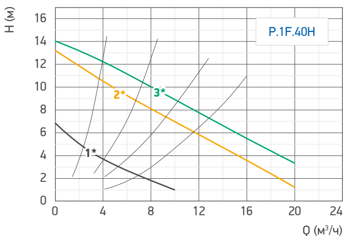
Гр. 72. Гидравлические характеристики насоса /P.1F.40H
