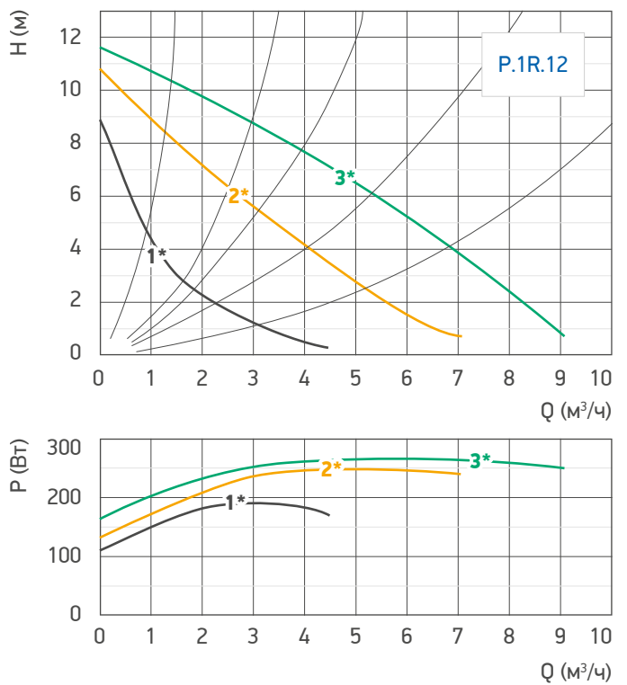
Гр. 70. Гидравлические характеристики насоса /P.1R.12
