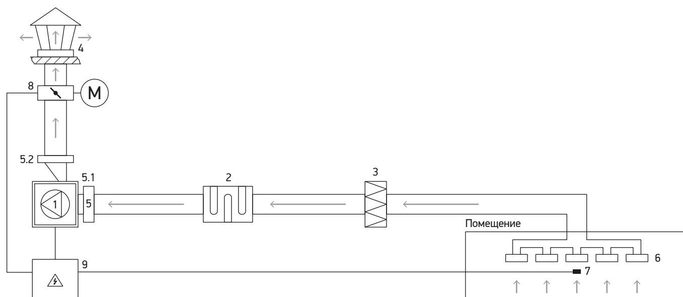
Схема 71. Рекомендованная схема монтажа вентиляторов /FPI
