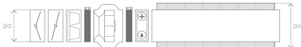
Схема 31. Габаритные размеры установок LM DUCT R
