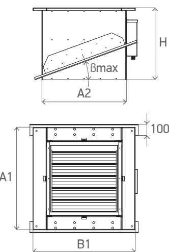
Табл. 53. Габаритные и присоединительные размеры монтажных стаканов /TSN.B, /TSN.N
