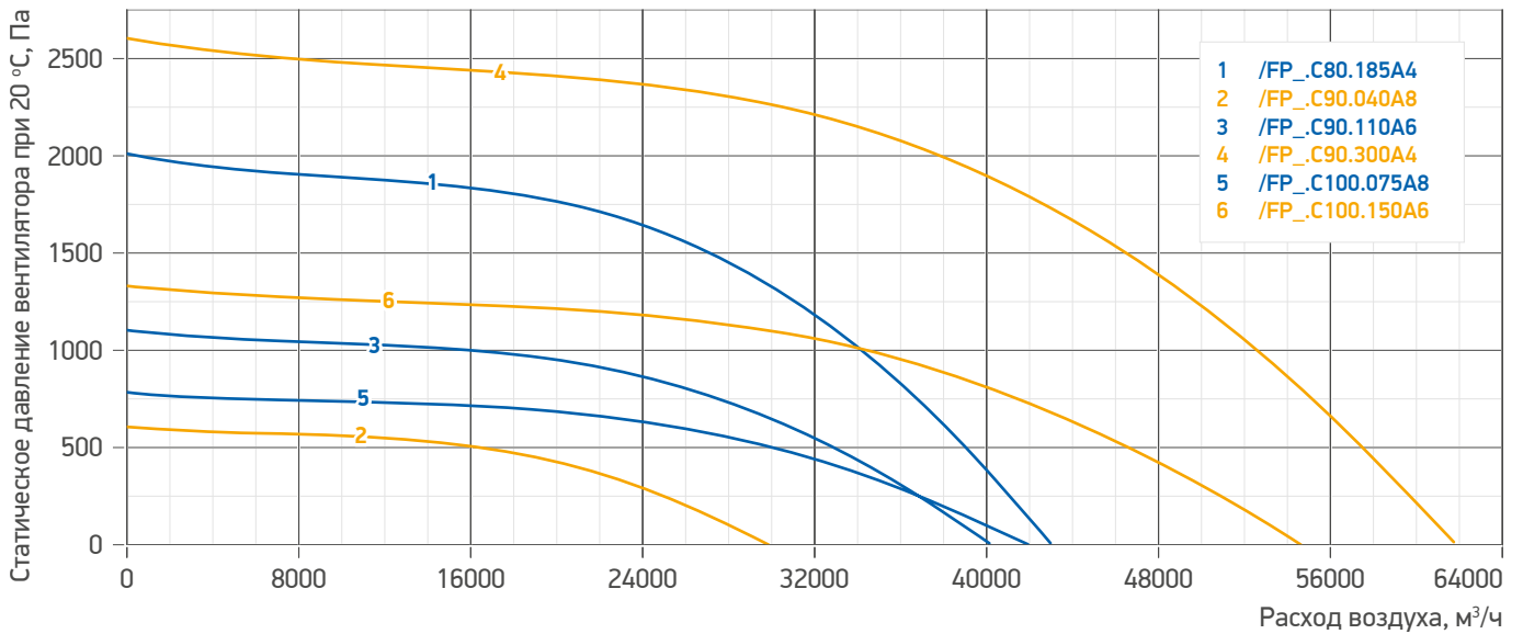
Гр. 44. Аэродинамические характеристики вентиляторов LM SAUGER /FB_
