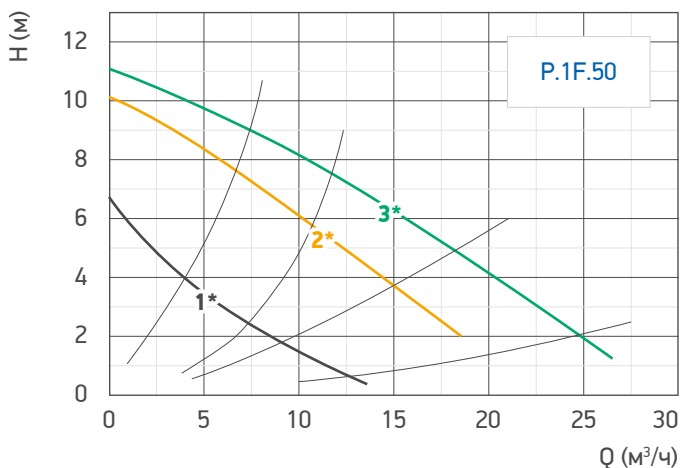
Гр. 73. Гидравлические характеристики насоса /P.1F.50
