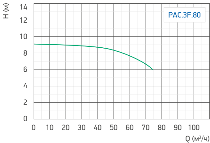
Гр. 87. Гидравлические характеристики насоса /PAC.3F.80
