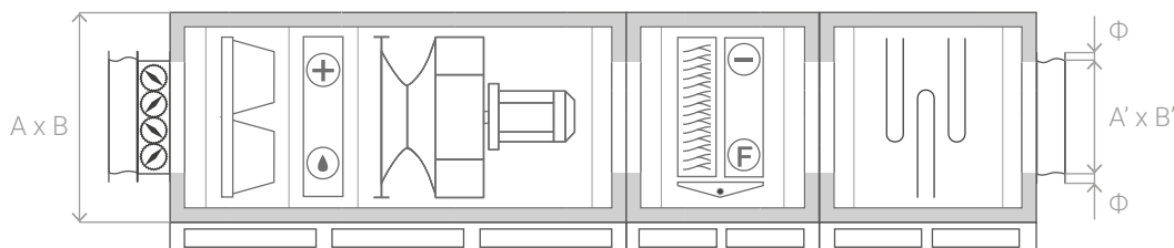
Табл. 61. Габаритные размеры и скорости воздуха в сечениях установок LM KERN 30
