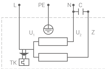
Схема 13. Схема B
