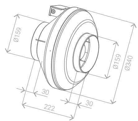
Схема 34. Вентилятор 160 /FBP.E22.2E
