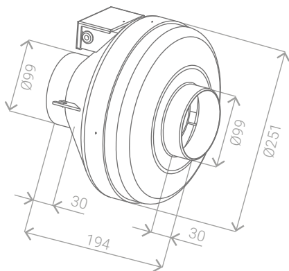
Схема 32. Вентилятор 100 /FBP.E19.2E
