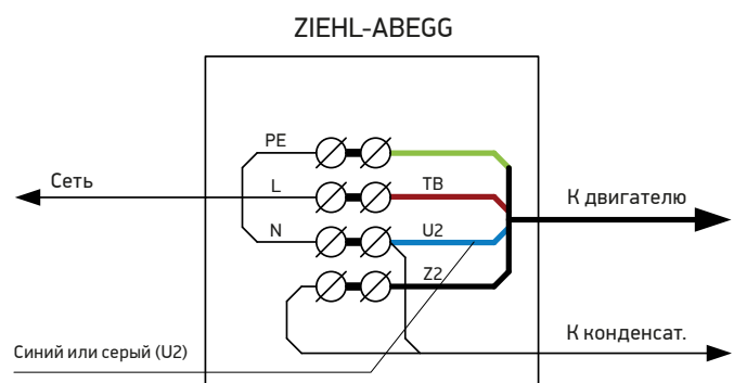
Схема 39. Монтажная схема подключения вентиляторов /FBP с мотор-колесом ZIEHL-ABEGG
