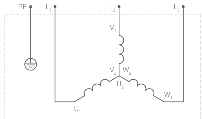
Схема 9. Схема С1
