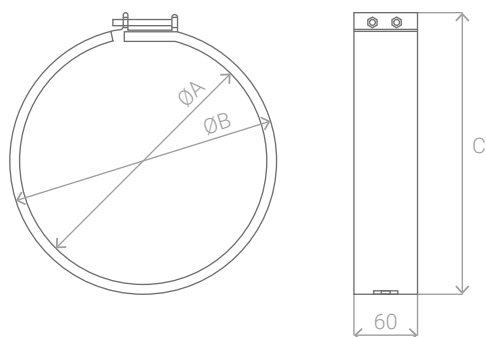
Схема 49. Габаритные размеры хомутов быстросъемных /Г.1
