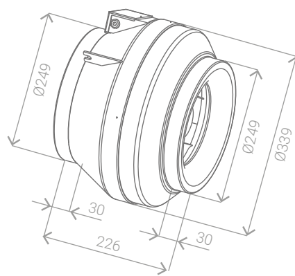
Схема 36. Вентилятор 250 /FBP.E25.2E
