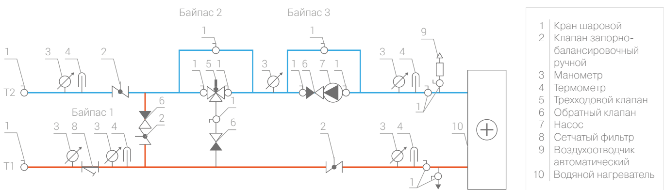
Схема 74. Рекомендованная схема обвязки водяного нагревателя
