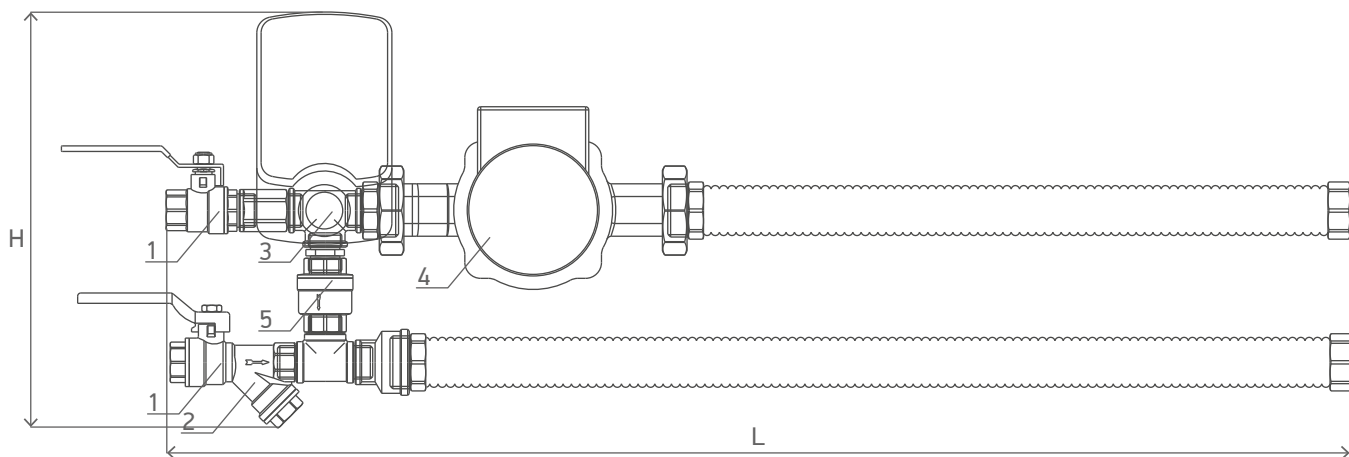
Схема 83. Смесительный узел /MUB_..._CP
