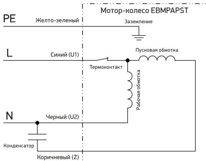
Схема 40. Принципиальная схема подключения вентиляторов /FBP с мотор-колесом EBMPAPST
