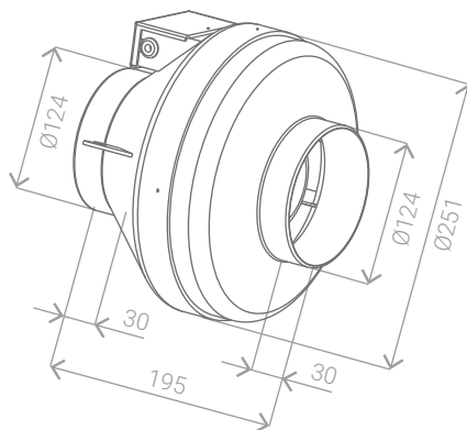
Схема 33. Вентилятор 125 /FBP.E19.2E
