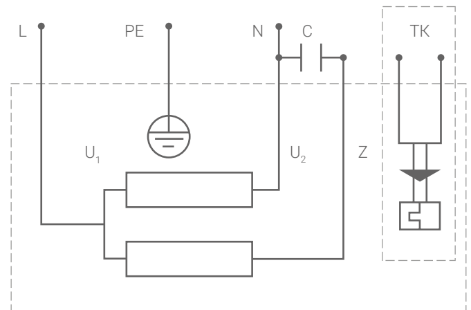
Схема 7. Схема В1
