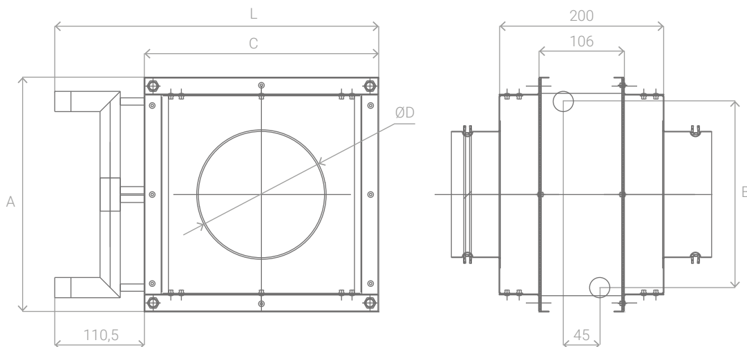
Схема 42. Габаритные размеры водяных нагревателей /HW
