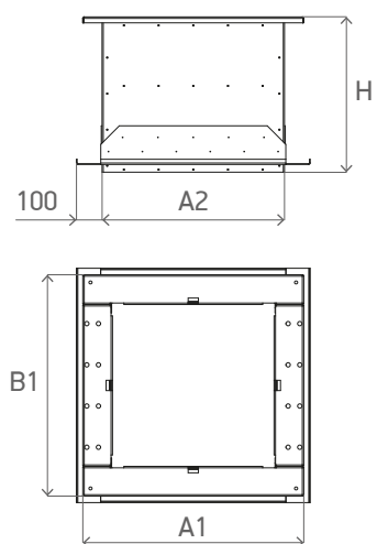
Табл. 53. Габаритные и присоединительные размеры монтажных стаканов /TSN.B, /TSN.N
