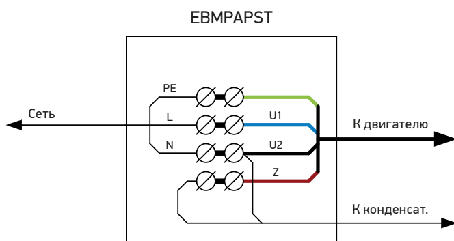
Схема 38. Монтажная схема подключения вентиляторов /FBP с мотор-колесом EBMPAPST
