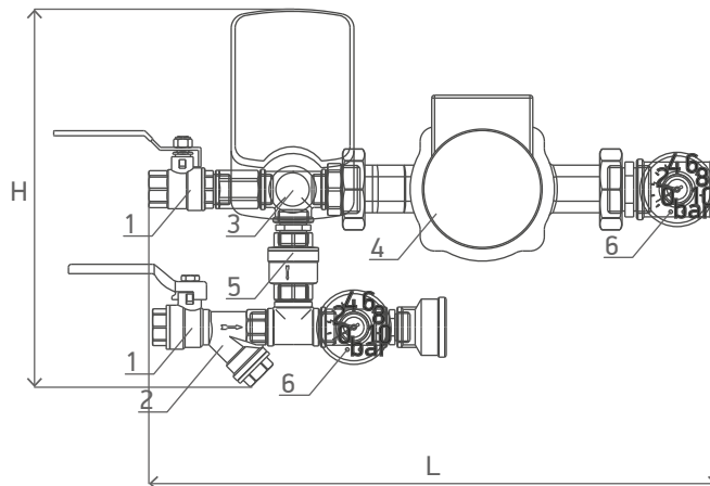
Схема 82. Смесительный узел /MUB_..._TM
