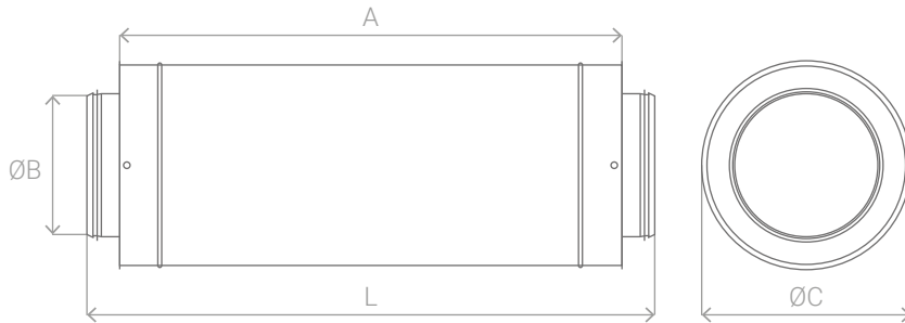
Схема 46. Габаритные размеры шумоглушителей /SP
