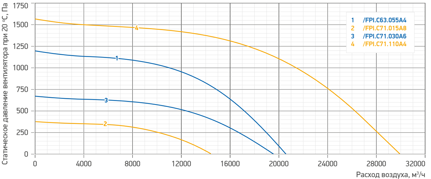
Гр. 47. Аэродинамические характеристики вентиляторов LM WURFEL /FPI (продолжение)
