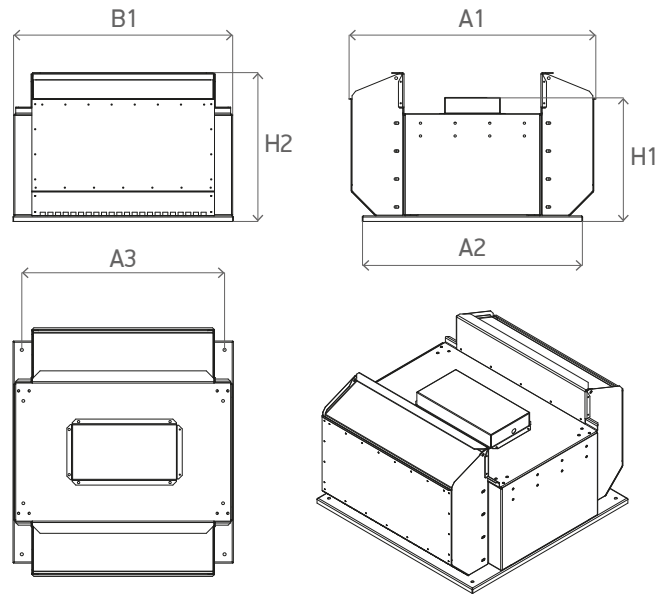
Схема 57. Габаритные характеристики вентиляторов /FBV
