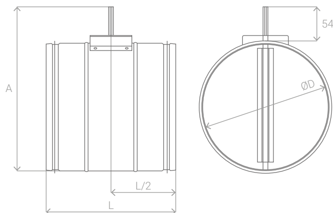
Схема 47. Габаритные размеры воздушных заслонок V.1
