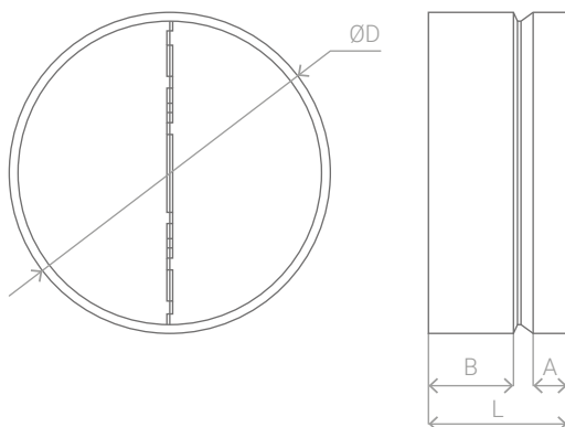
Схема 48. Габаритные размеры обратных клапанов /VO.1
