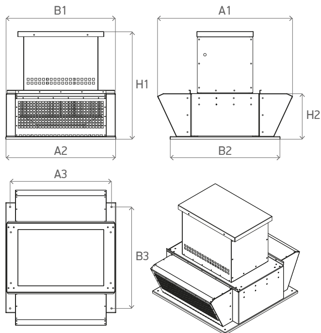
Схема 54. Габаритные характеристики вентиляторов /FPH
