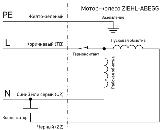
Схема 41. Принципиальная схема подключения вентиляторов /FBP с мотор-колесом ZIEHL-ABEGG
