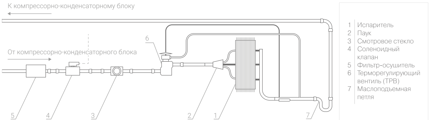
Схема 76. Схема обвязки контура испарителя
