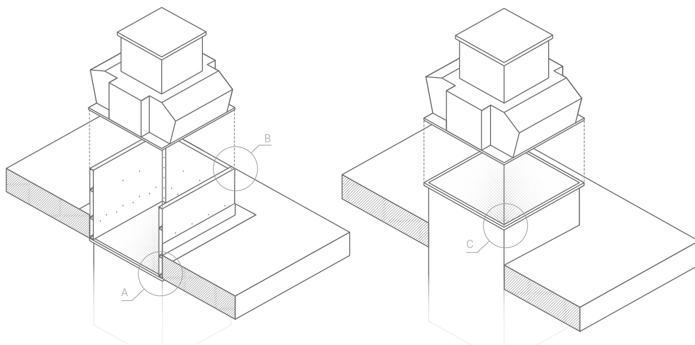
Схема 53. Узел крепления монтажного стакана к воздуховоду, вентилятора к монтажному стакану
