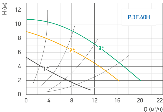
Гр. 74. Гидравлические характеристики насоса /P.3F.40H
