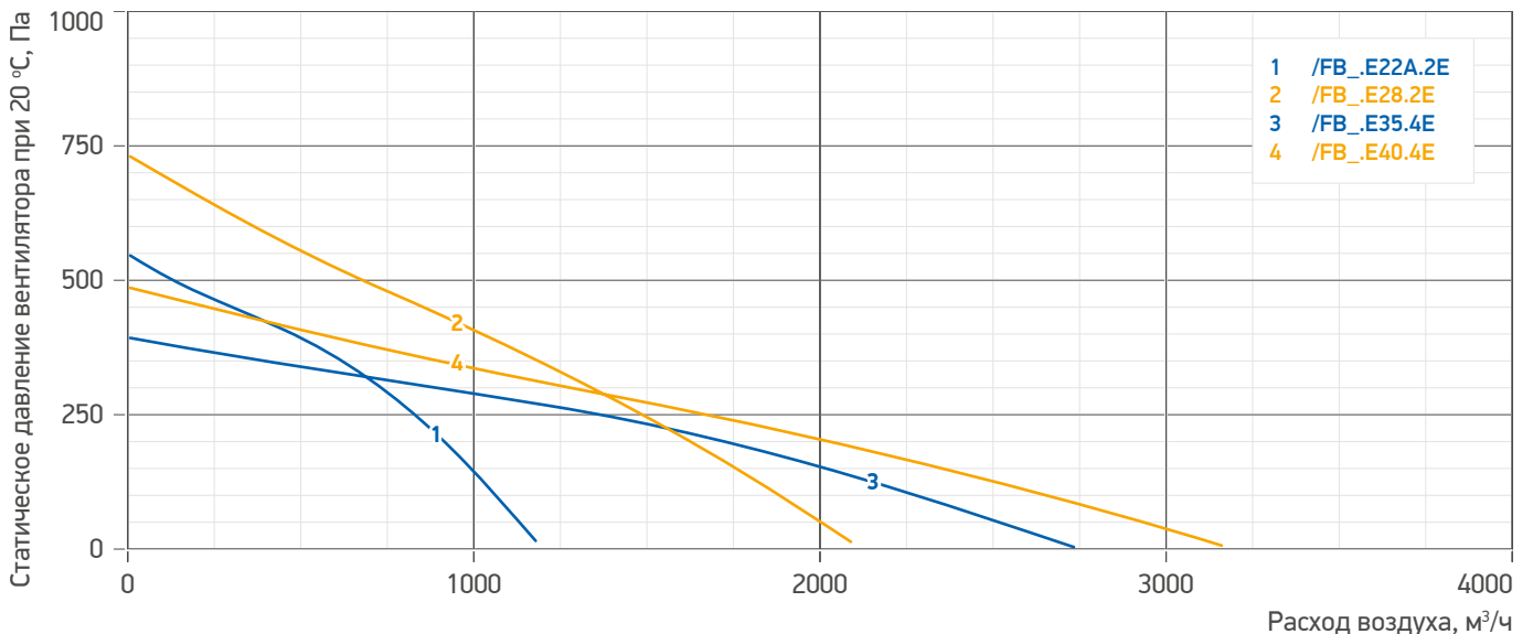
Гр. 45. Аэродинамические характеристики вентиляторов LM SAUGER /FB_ (продолжение)
