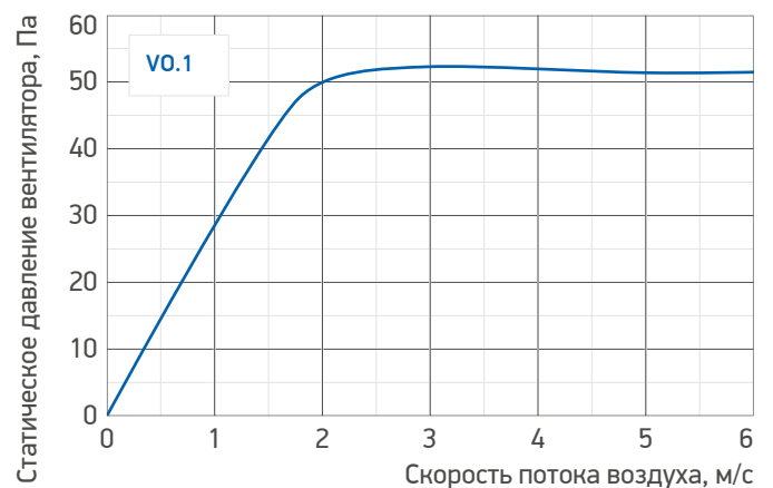
Гр. 38. Аэродинамические характеристики обратных клапанов /VO.1
