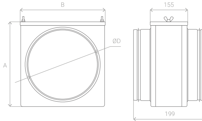
Схема 45. Габаритные размеры фильтров кассетных /EG
