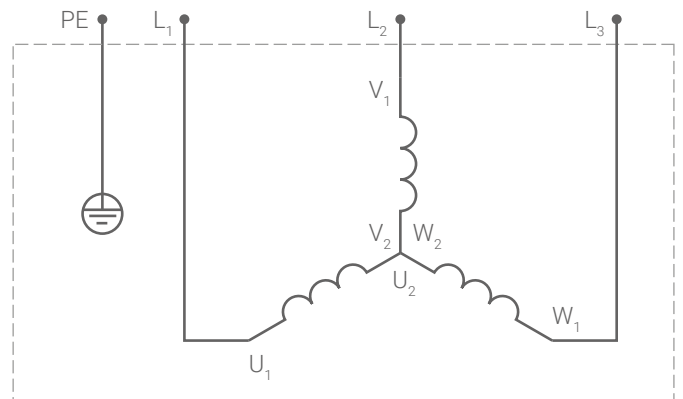
Схема 17. Схема C1
