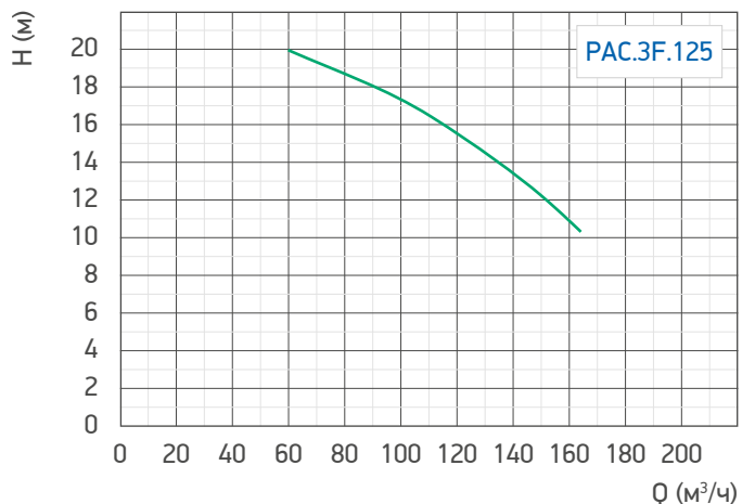
Гр. 88. Гидравлические характеристики насоса /PAC.3F.125
