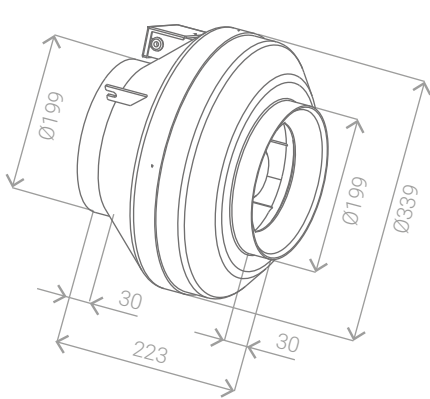
Схема 35. Вентилятор 200 /FBP.E22A.2E
