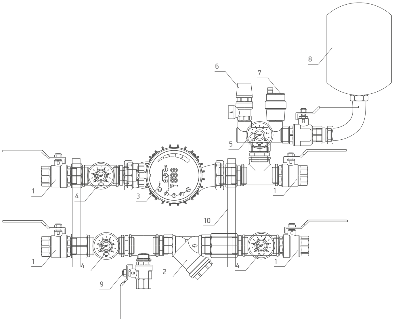
Схема 85. Смесительный узел /MUG_..._EC
