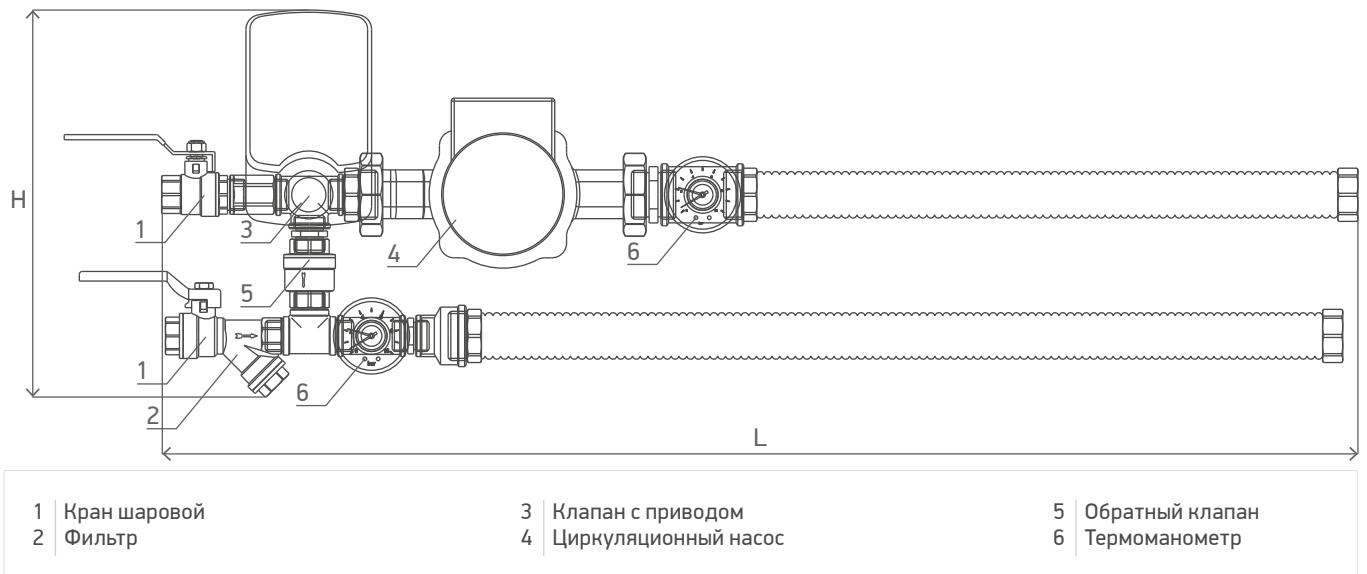
Схема 84. Смесительный узел /MUB...CP.TM
