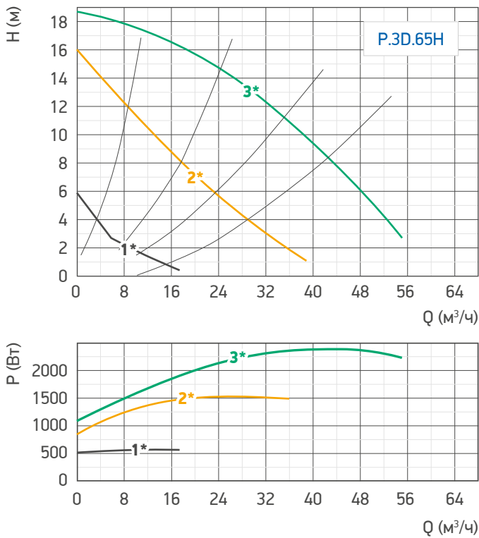
Гр. 81. Гидравлические характеристики насоса /P.3D.65H
