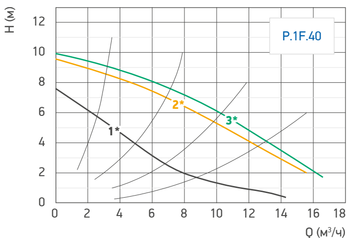
Гр. 71. Гидравлические характеристики насоса /P.1F.40
