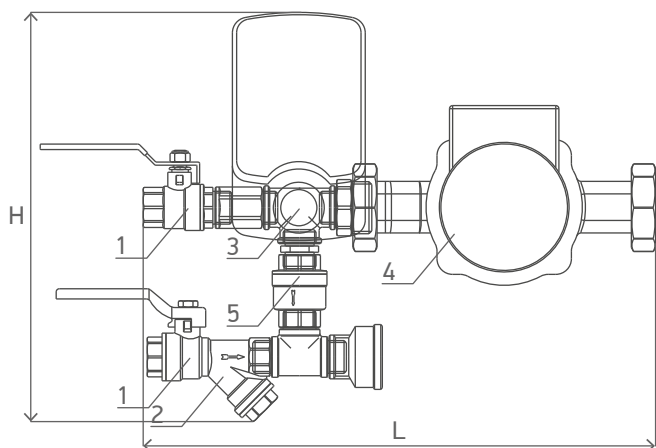
Схема 81. Смесительный узел /MUB_..._.
